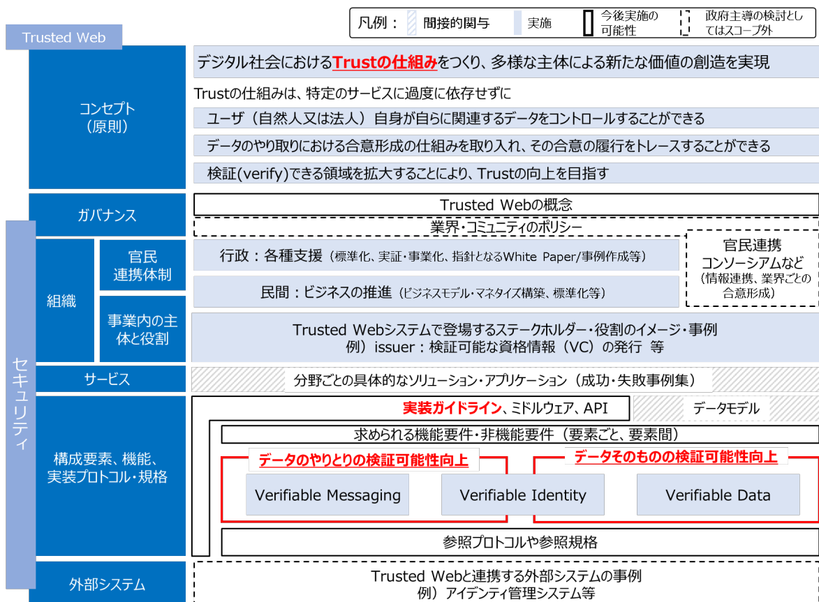
図 1-2 Trusted Web における全体像
