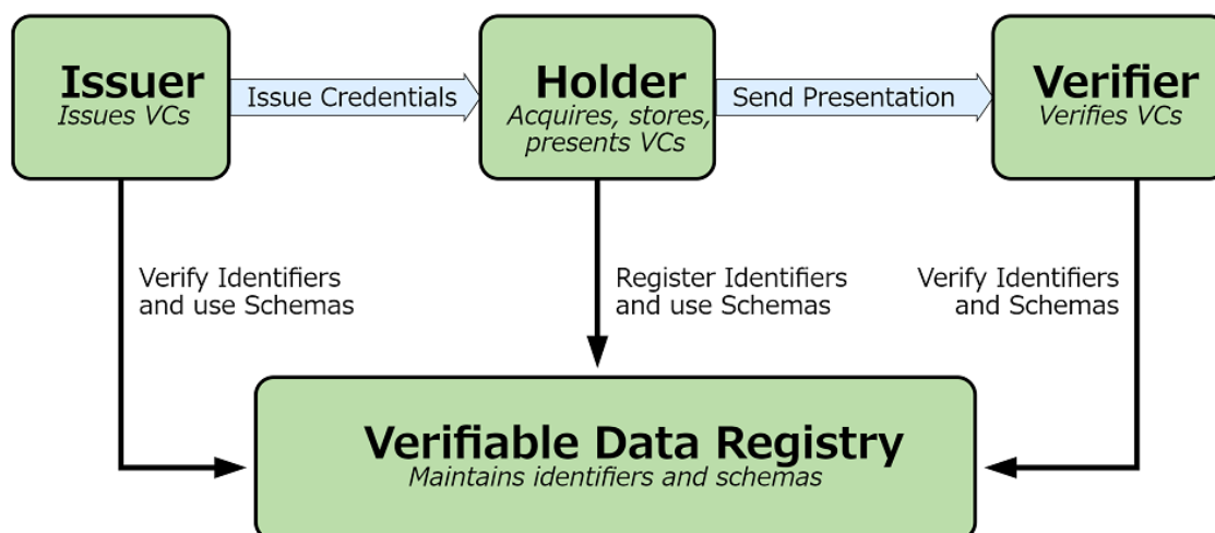
図 6-3 Verifiable Credentials Data Model における基本的な役割と情報の流れ 22
