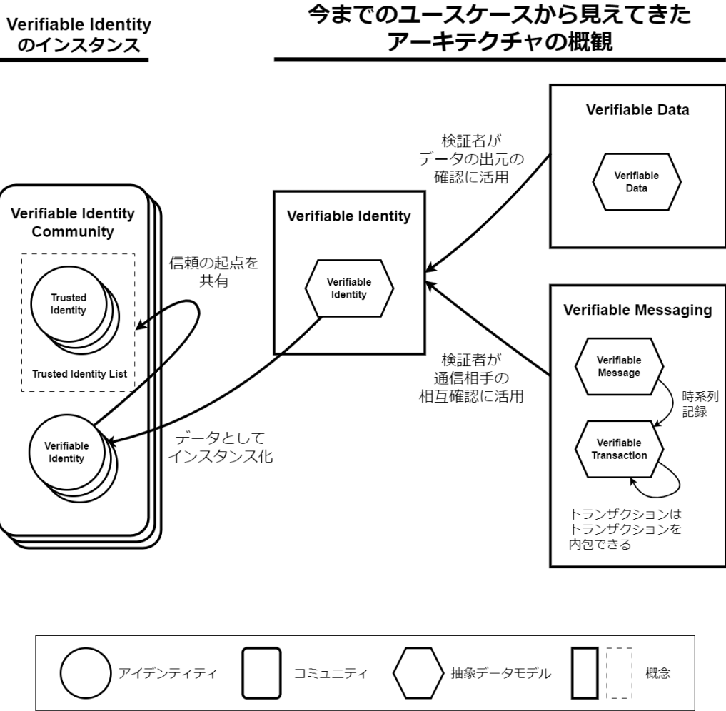
図 3-1 Trusted Web アーキテクチャ概観
